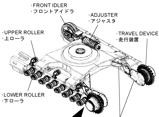
・TRAVEL PIPING COVER ・走行配管カバー
