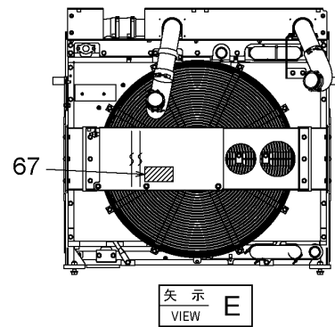
Fan drive inside ファンドライブ内側
