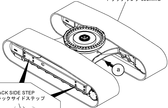
TRACK LINK 600mmG トラックリンク 600mmG
