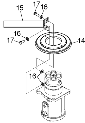
詳細 B DETAIL B
