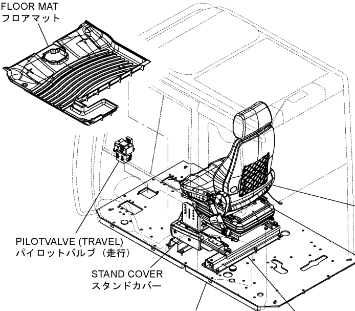
AIR SUSPENSION SEAT PARTS (WITH HEATER) (KAB) エアサスペンションシート用品 (ヒータ付) (KAB) ・ AIR SUSPENSION SEAT (WITH HEATER) (KAB) ・ エアサスペンションシート (ヒータ付) (KAB)
