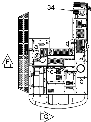
Upperstructure Top 旋回体上面
