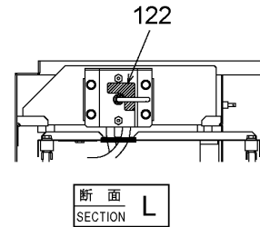
Battery disconnect switch バッテリーディスコネクトスイッチ
