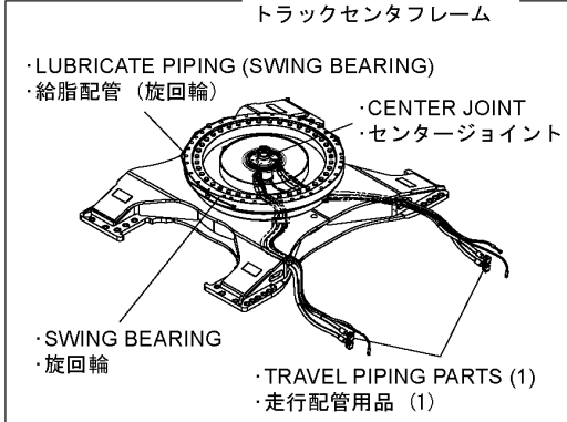
TRACK CENTER FRAME トラックセンタフレーム
