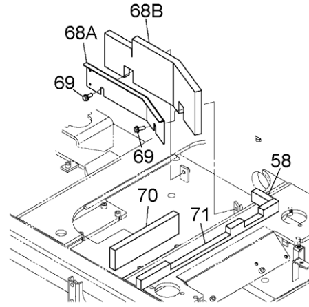
詳細 A DETAIL A
