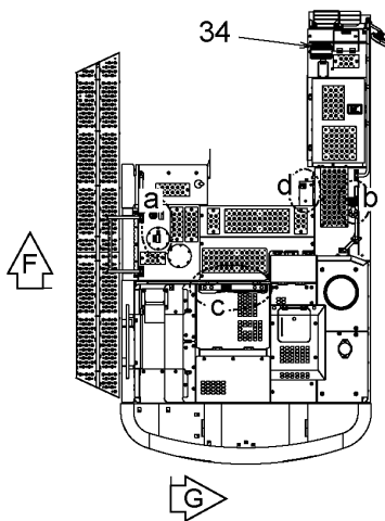
Upperstructure Top 旋回体上面
